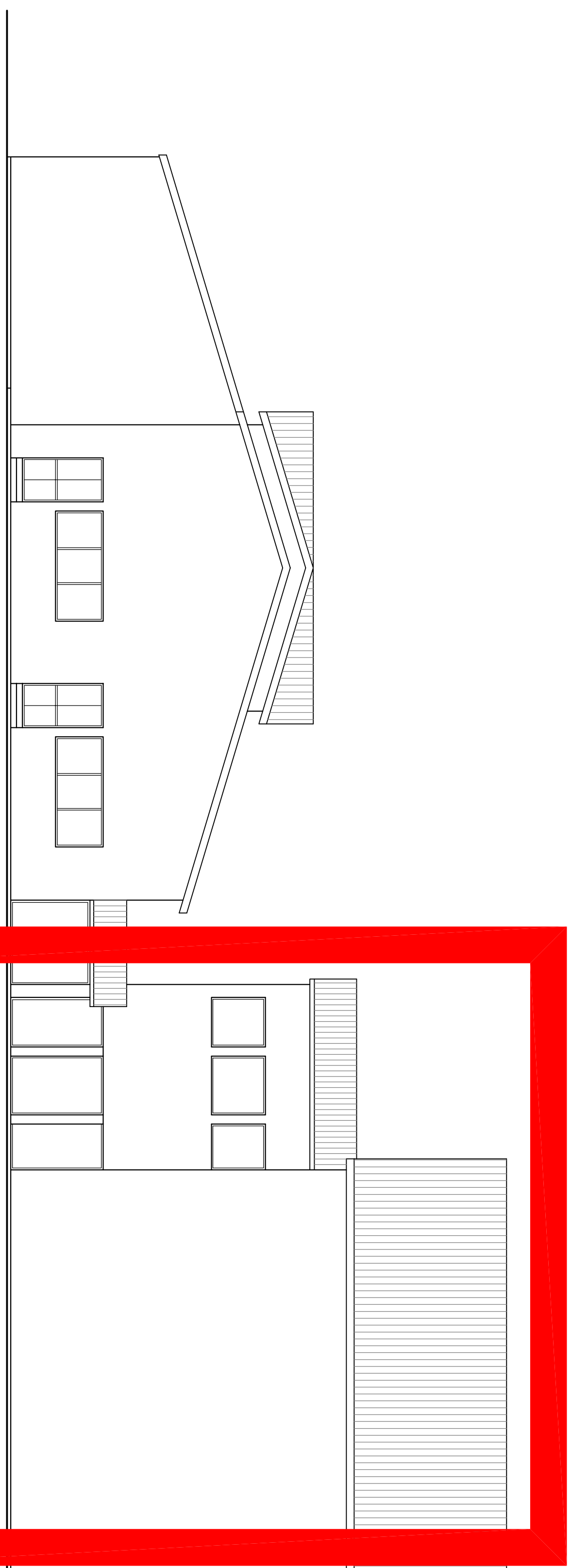
PROSPETTO -B-
