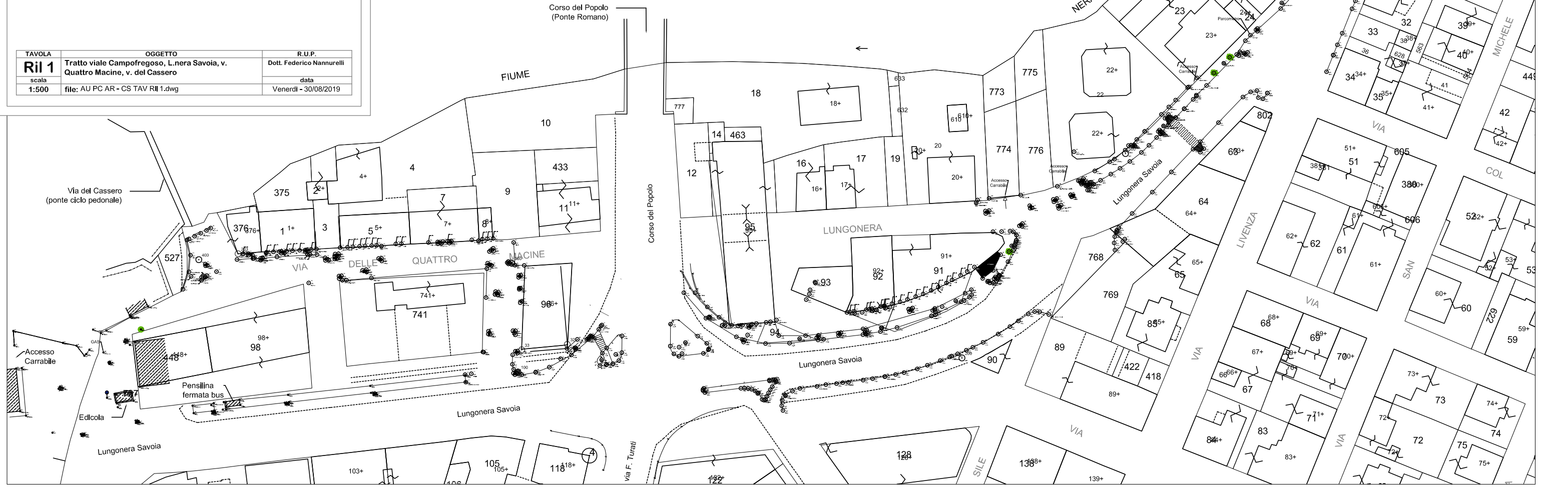
Stralcio rilievo incrocio Lungonera Savoia - P.le Garibaldi - via G. di Vitalone
