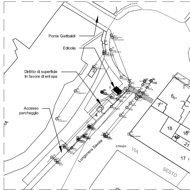
Stralcio rilievo incrocio Lungonera Savoia - P.le Garibaldi - via G. di Vitalone
